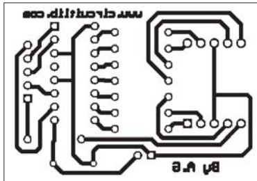
PCB - 1:1
